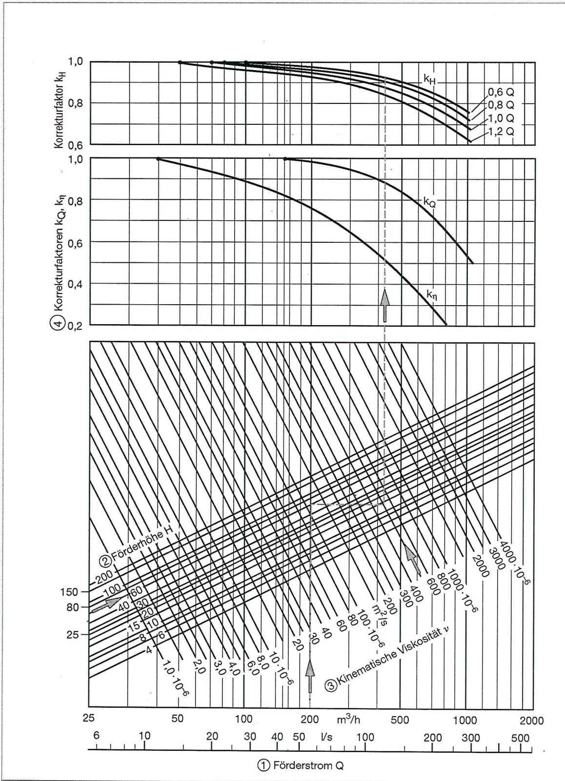
Bild 49: Ermittlung der Korrekturfaktoren k nach Standards of Hydraulic Institute. Eingetragenes Beispiel für Q = 200 m^3/h , H = 57,5 m , \nu = 500 \cdot 10^{-6} m^2/s
